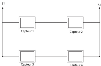
Figure 1 – Capteur à distance – Câblage en parallèle Remarques importantes concernant le câblage
