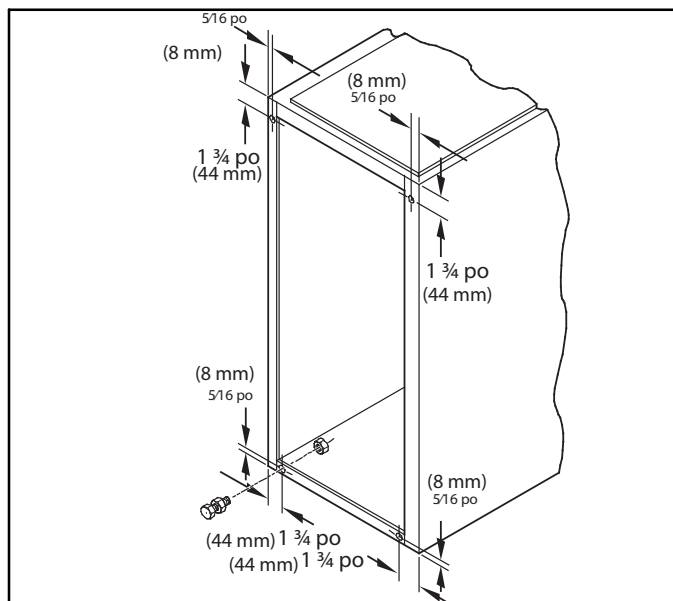
Figure 22 – Pattes de mise à niveau
