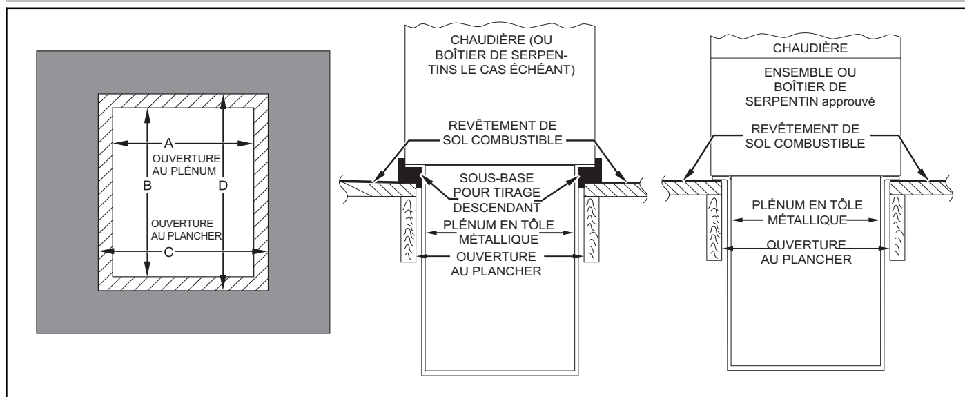
Figure 20 – Installation sur revêtement de plancher combustible
