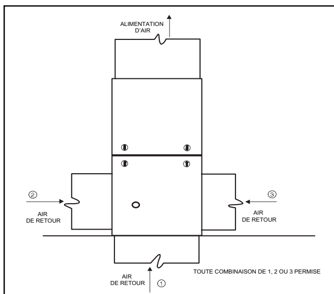
Figure 25 – Configurations et restrictions des conduits de retour d'air ascendant
