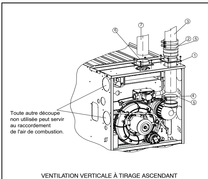
Figure 42 – Configurations à tirage ascendant (l'apparence peut varier) Consultez les « Remarques concernant les options de ventilation ».
