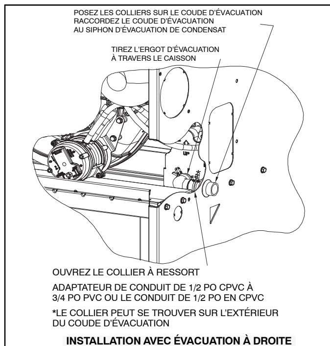
Figure 13 – Exemple de fixation au tuyau d'évacuation sur place
