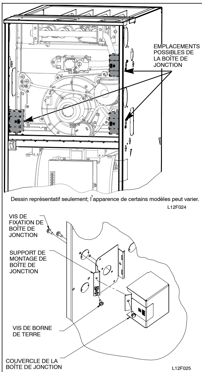
Figure 33 – Installation d'une boîte de jonction (le cas échéant)
