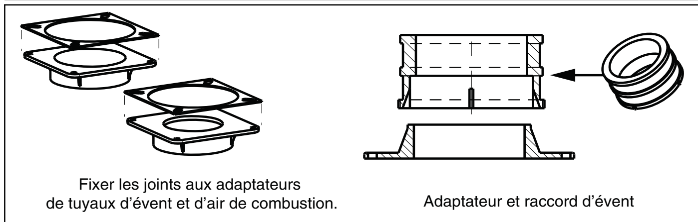
Figure 39 – Raccord d'évent et adaptateur avec joints
