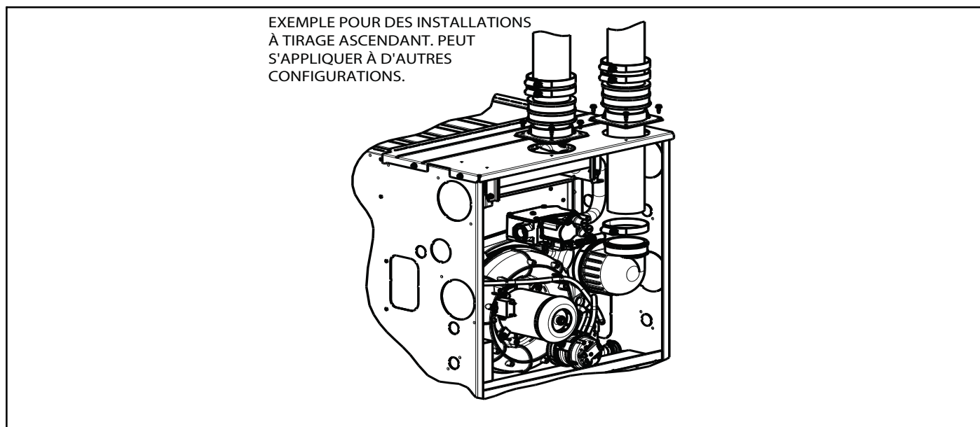
Figure 41 – Exemple de raccordement de tuyau d'air pour des systèmes de ventilation en polypropylène
