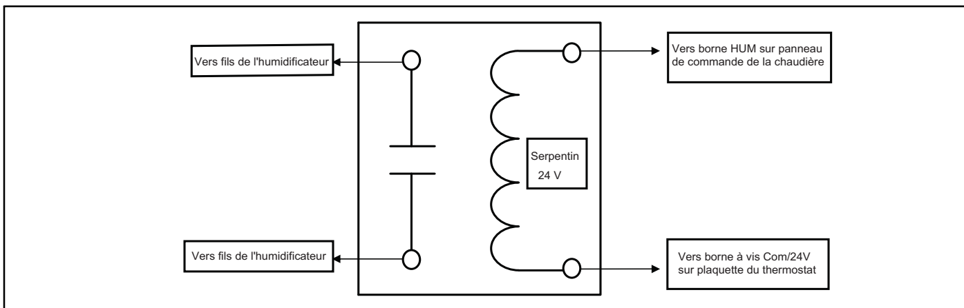
Figure 35 – Relais d'isolation pour humidificateurs, fourni sur place, avec bloc d'alimentation interne
