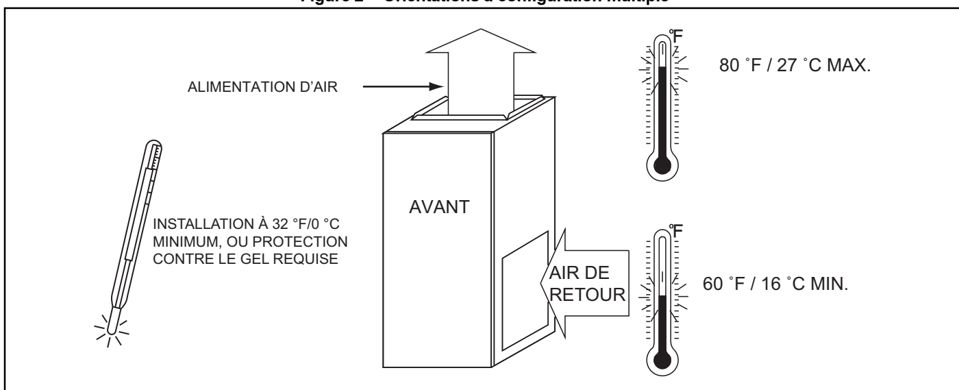
Figure 3 – Protection contre le gel et température de l'air de retour
