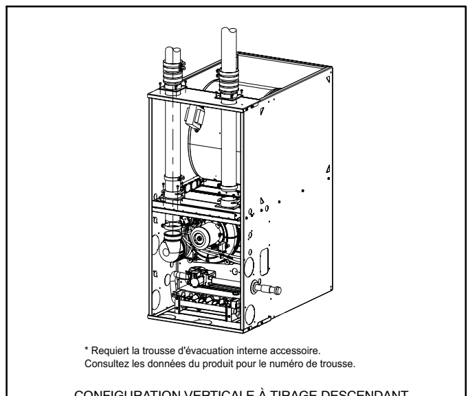
Figure 43 – Configurations à tirage descendant (l'apparence peut varier). Voir les « Remarques concernant les options de ventilation ».
