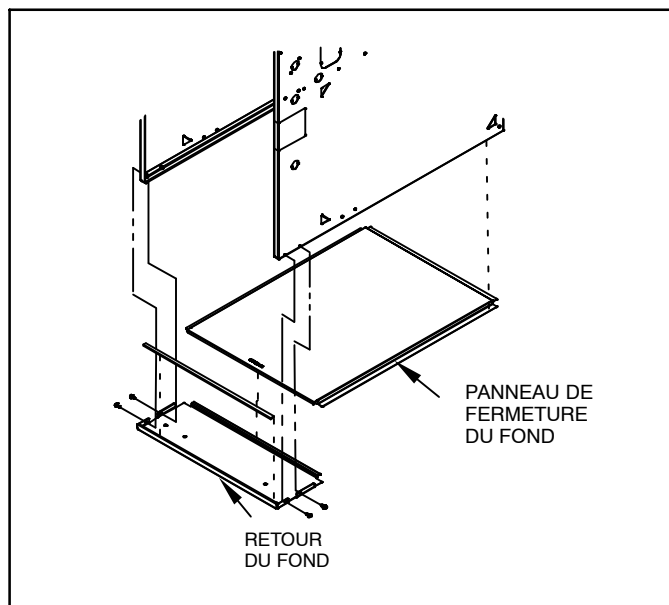
Figure 23 – Retrait du panneau de fermeture du fond
