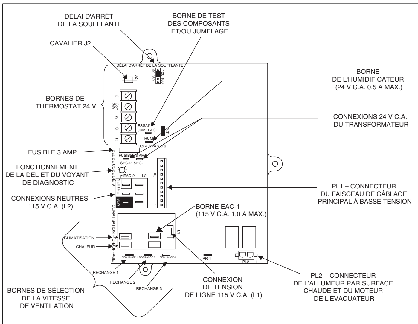
Figure 37 – Exemple de panneau de commande de chaudière à un étage
