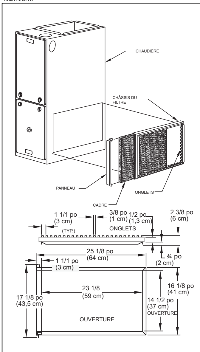
Figure 18 – Support de filtre latéral
