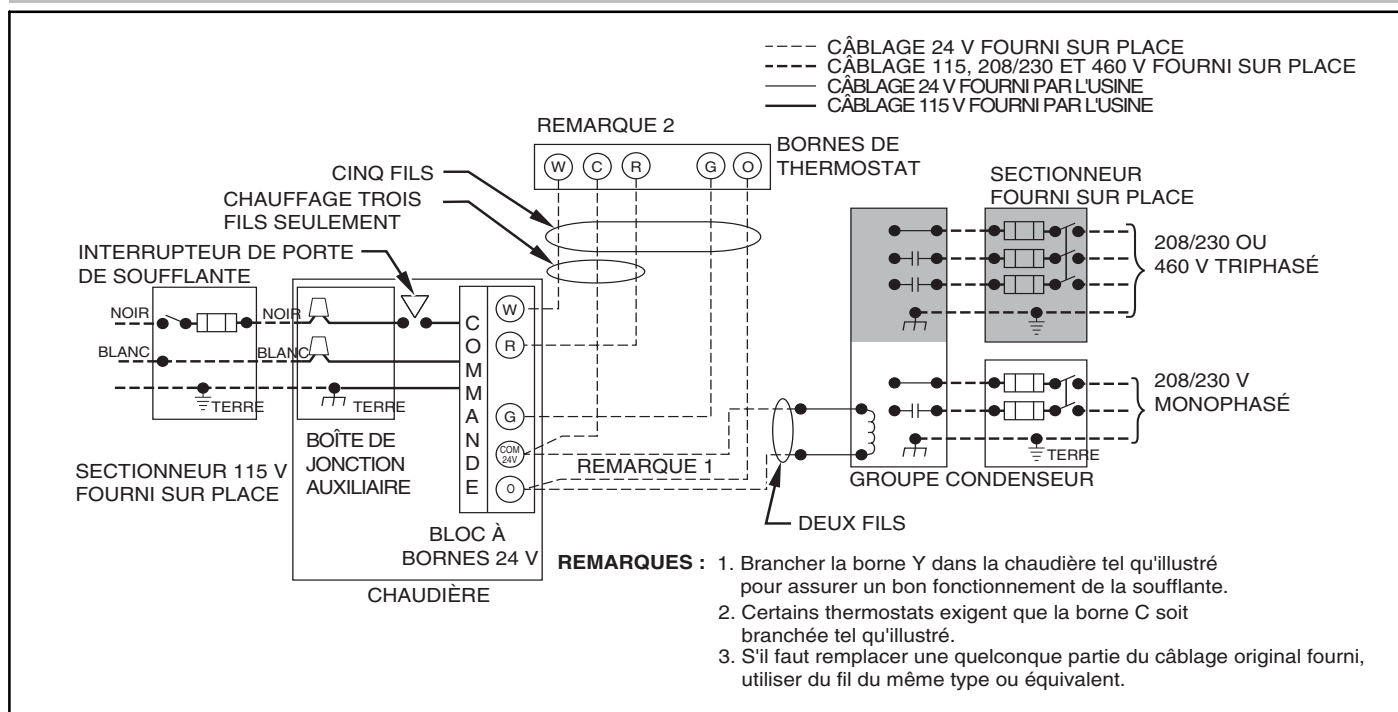
Figure 36 – Schéma de câblage type d'un appareil à un étage
