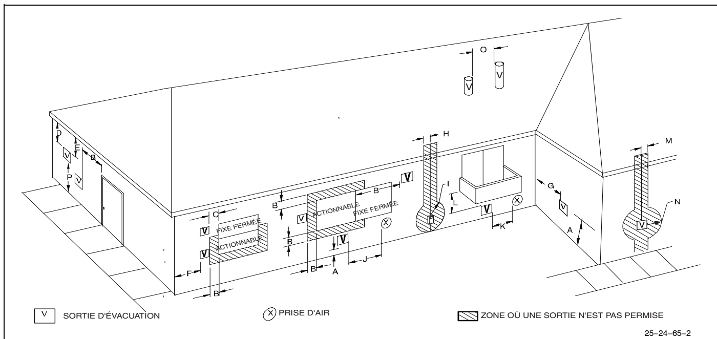
Figure 48 – Dégagement des terminaisons d'évent de système à ventilation directe
