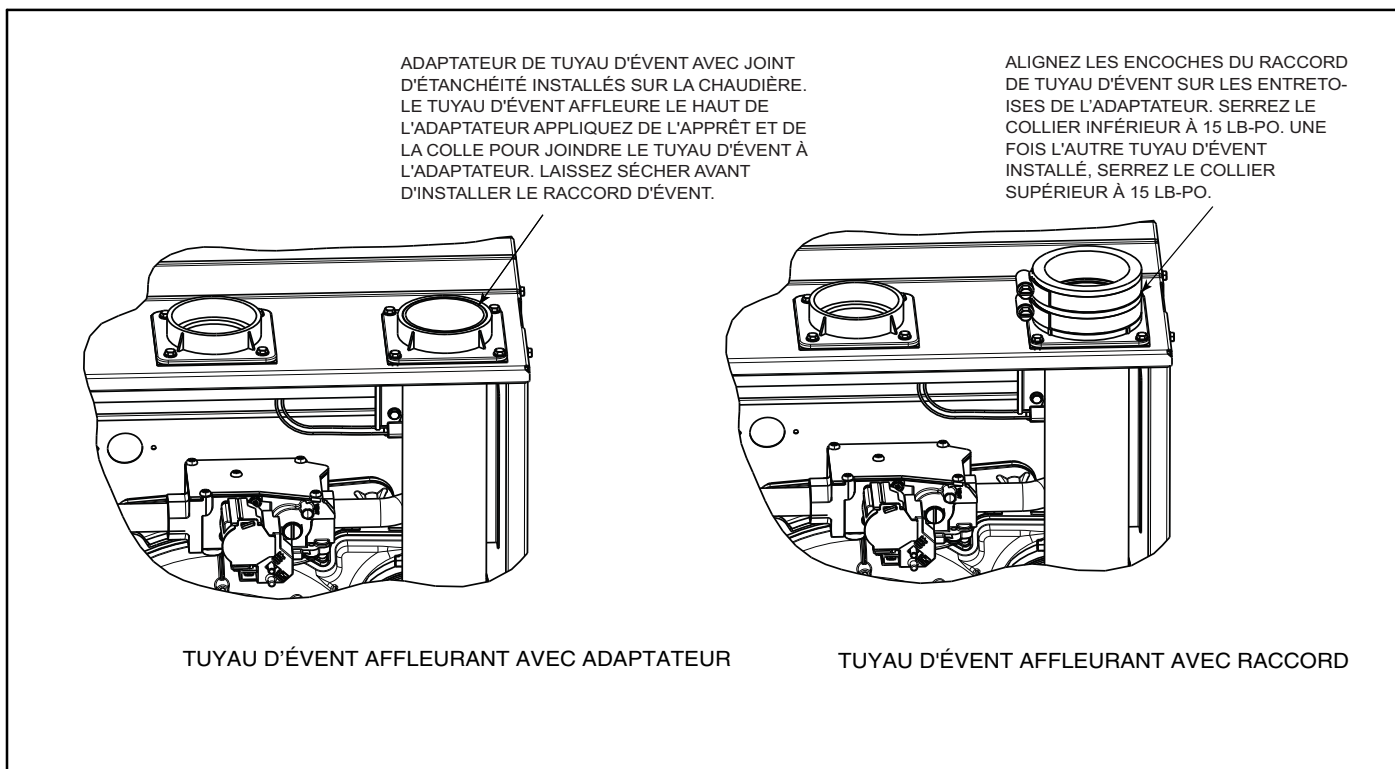
Figure 46 – Tuyau d'évent affleurant avec adaptateur
