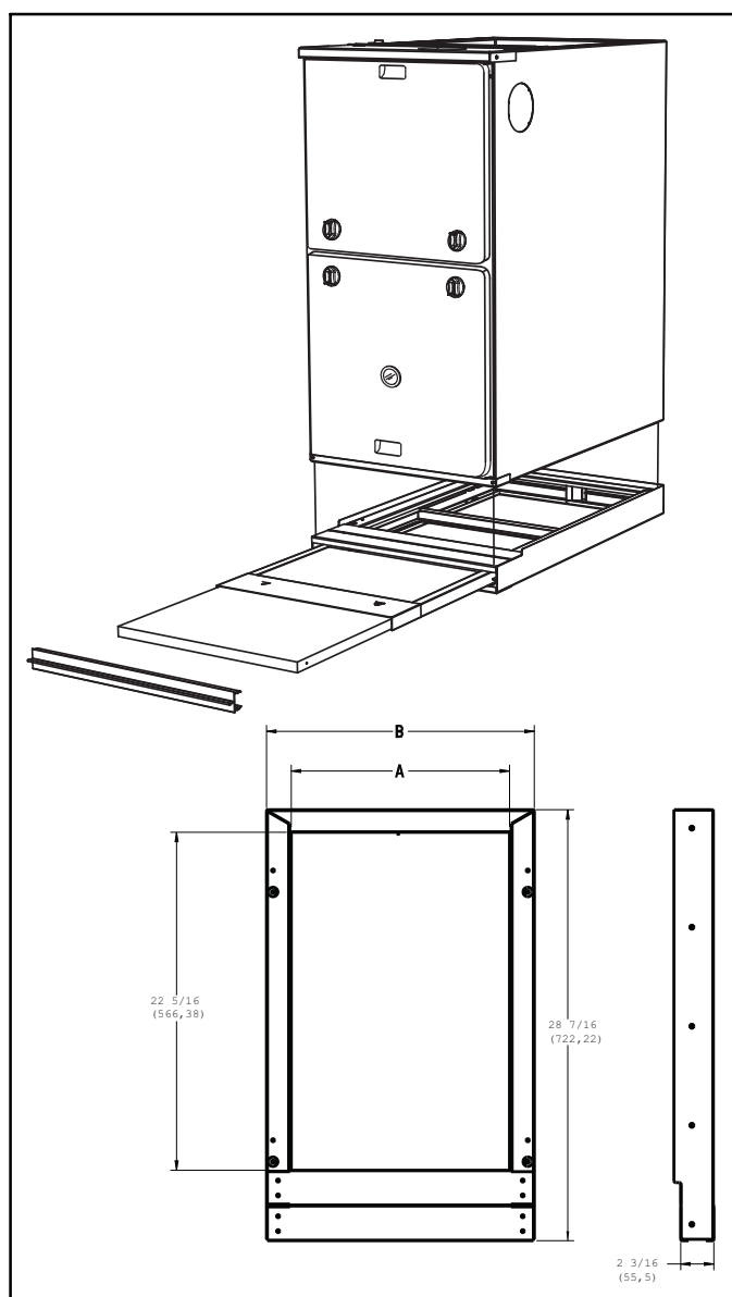
Figure 19 – Filtre du fond
