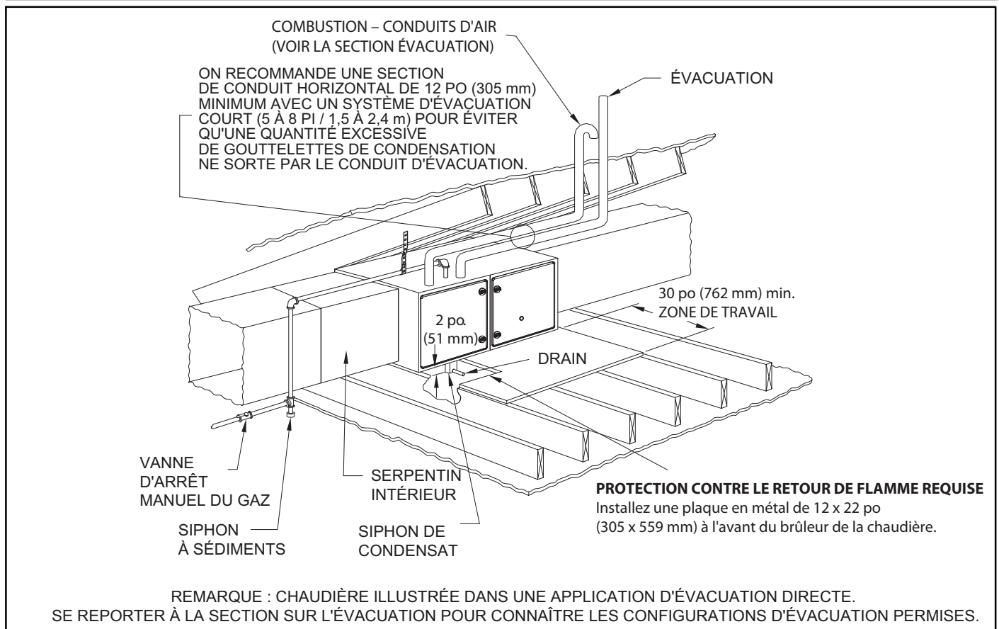
Figure 28 – Plateforme de travail pour installation dans le grenier
