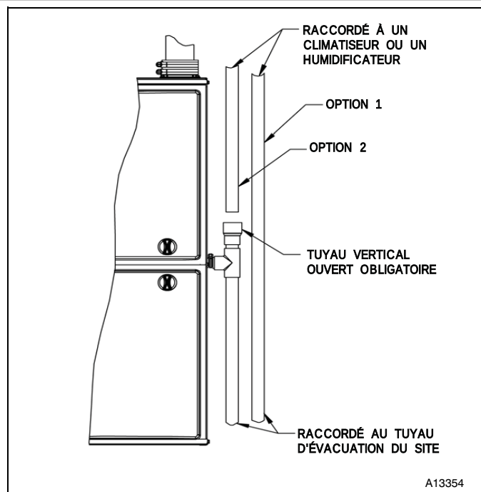
Figure 13 – Exemple de fixation au tuyau d'évacuation sur place
