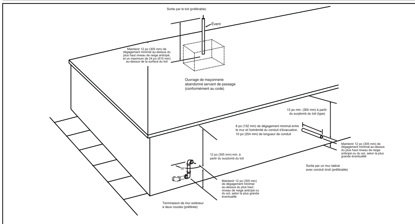
Figure 51 – Terminaison d'évent pour système à ventilation non directe et à air de combustion ventilé
