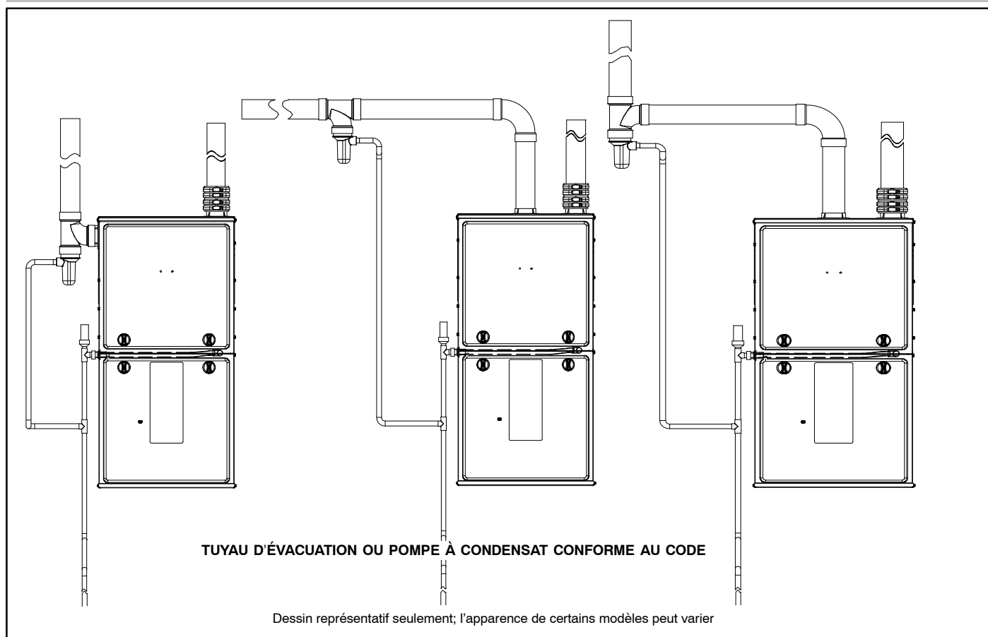
Figure 54 – Siphon de condensat d'air de combustion optionnel
