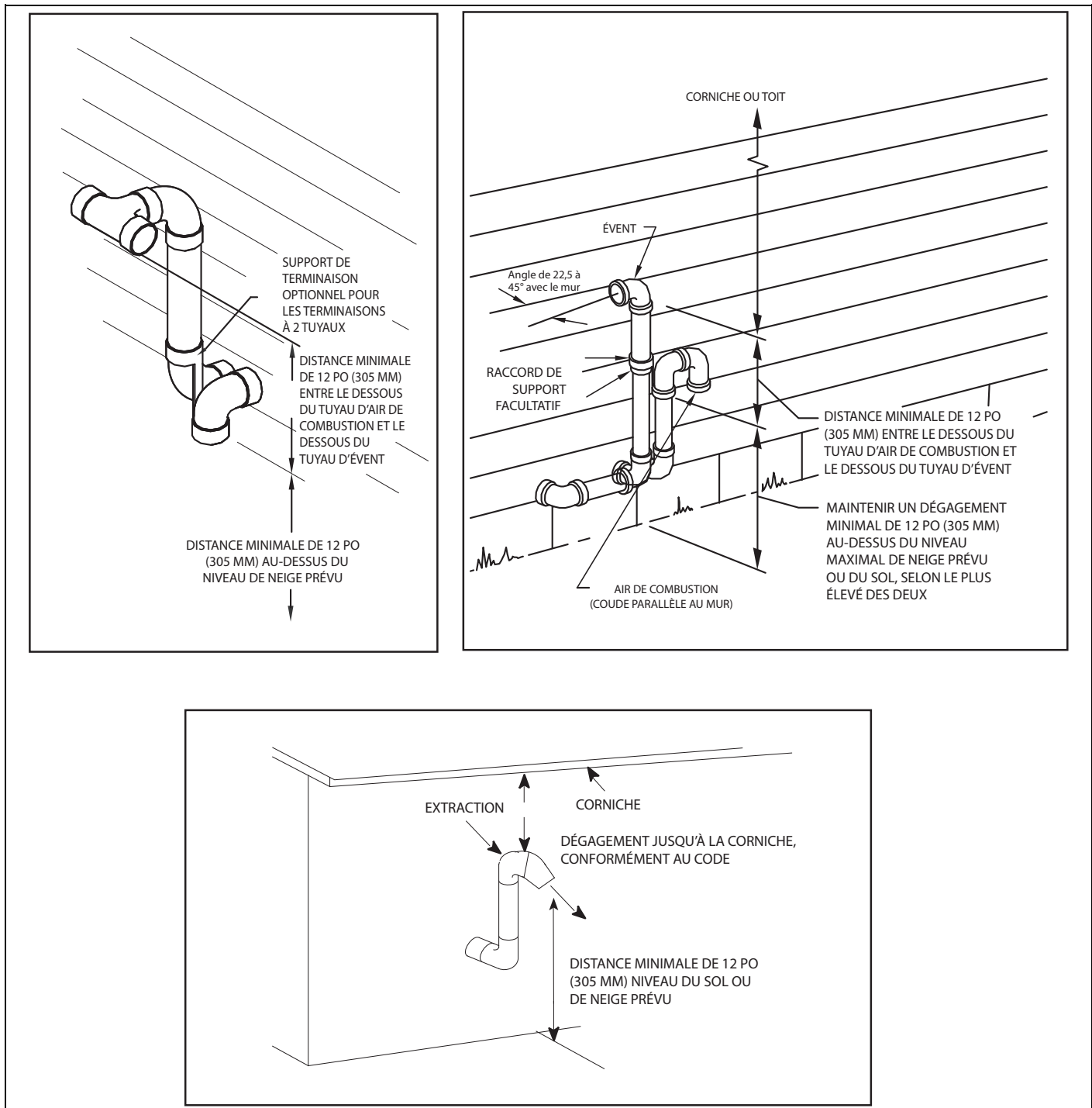
Figure 52 – Termination d'évent pour l'Alberta et la Saskatchewan
