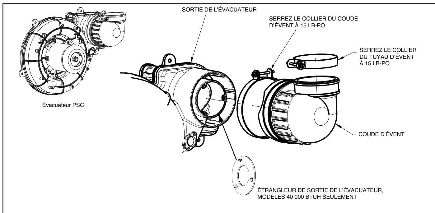
Figure 40 – Coude d'évent d'évacuateur
