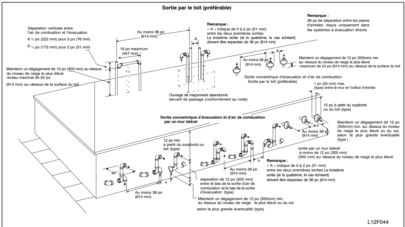
Figure 50 – Terminaisons de tuyaux d'air de combustion et d'évent pour système à ventilation directe (deux tuyaux)
