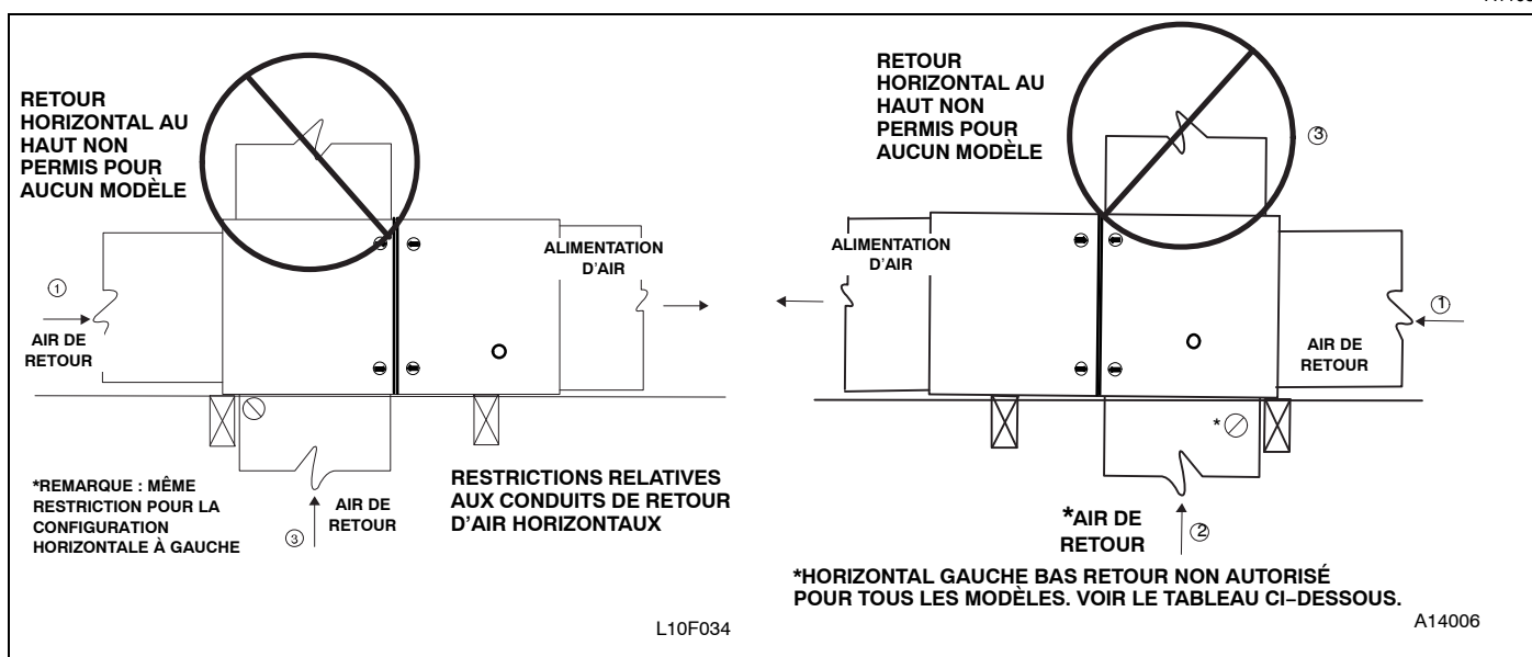
Figure 27 – Configurations et restrictions des conduits de retour d'air horizontaux
