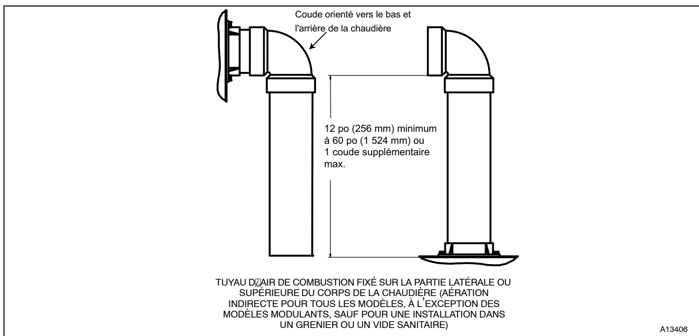
Figure 47 – Fixation du tuyau d'air de combustion
