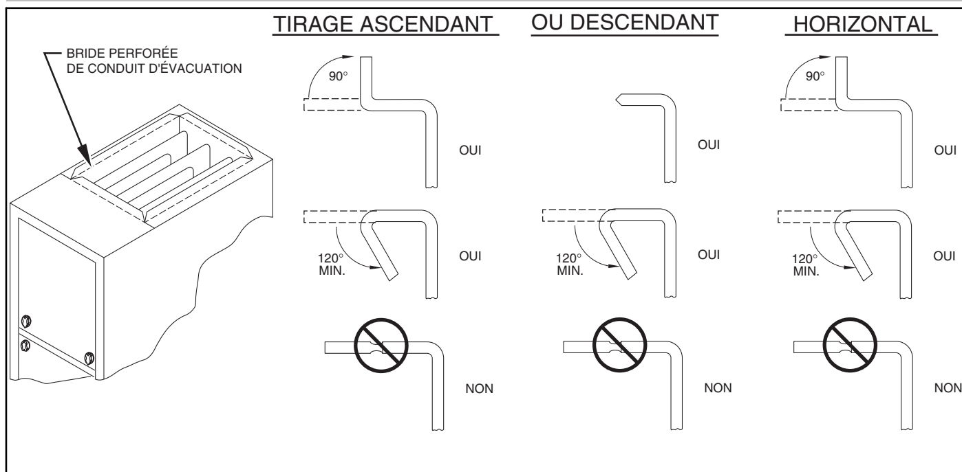
Figure 21 – Brides d'attache du conduit
