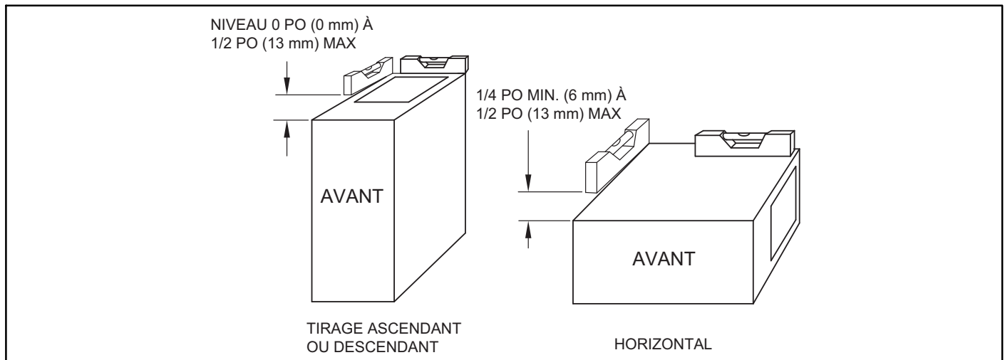
Figure 24 – Exigences d'inclinaison de la chaudière
