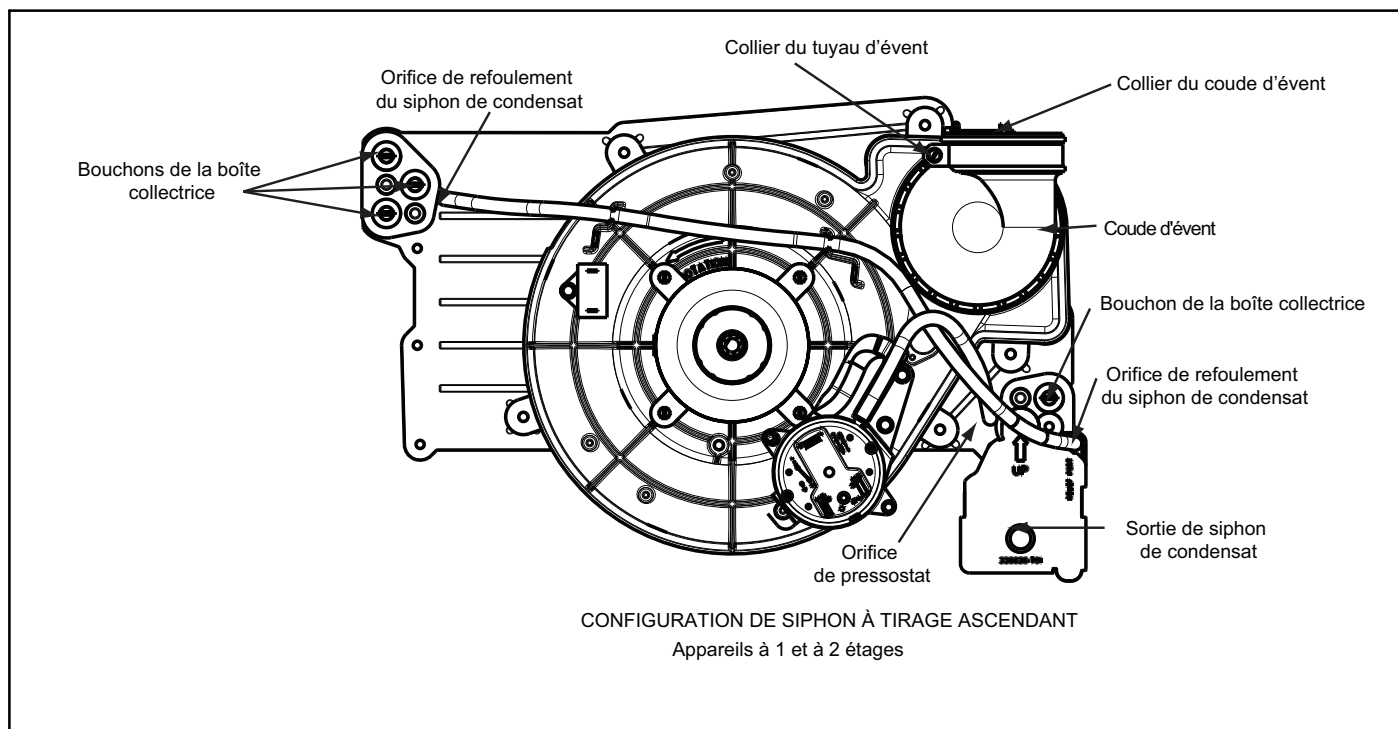
Figure 8 – Configuration de siphon à tirage ascendant (l'apparence peut varier)
