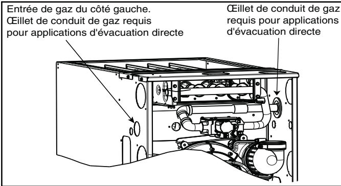
Figure 31 – Entrée de gaz
