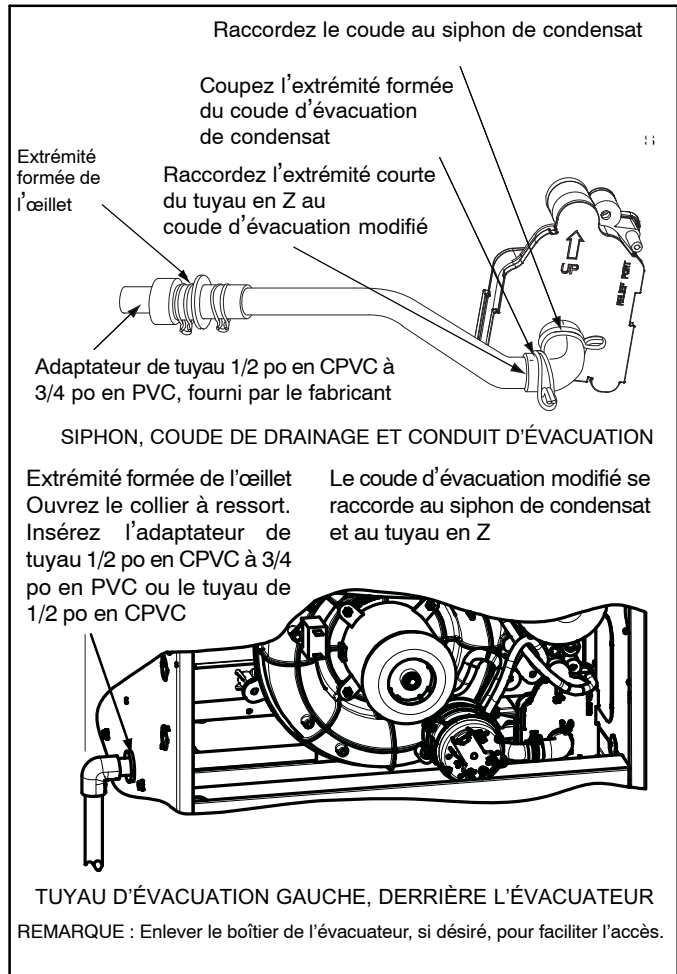
Figure 17 – Raccordement et acheminement du siphon d'évacuation (l'apparence peut varier)
