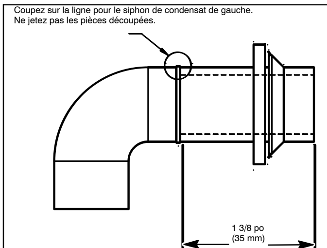
Figure 15 – Modification du coude de drainage en caoutchouc
