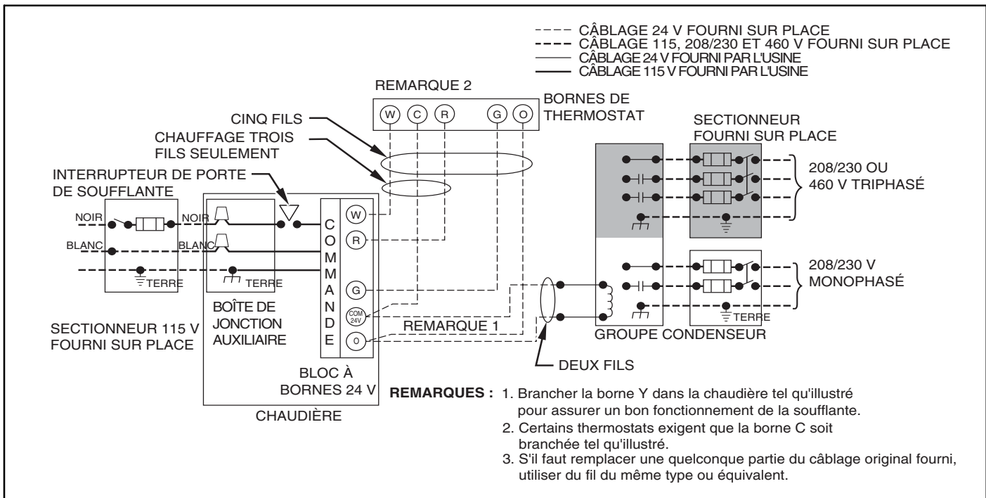
Figure 36 – Schéma de câblage type d'un appareil à un étage
