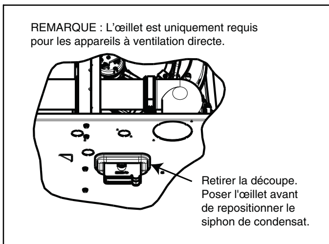
Figure 16 – Œillet de siphon d'évacuation horizontal
