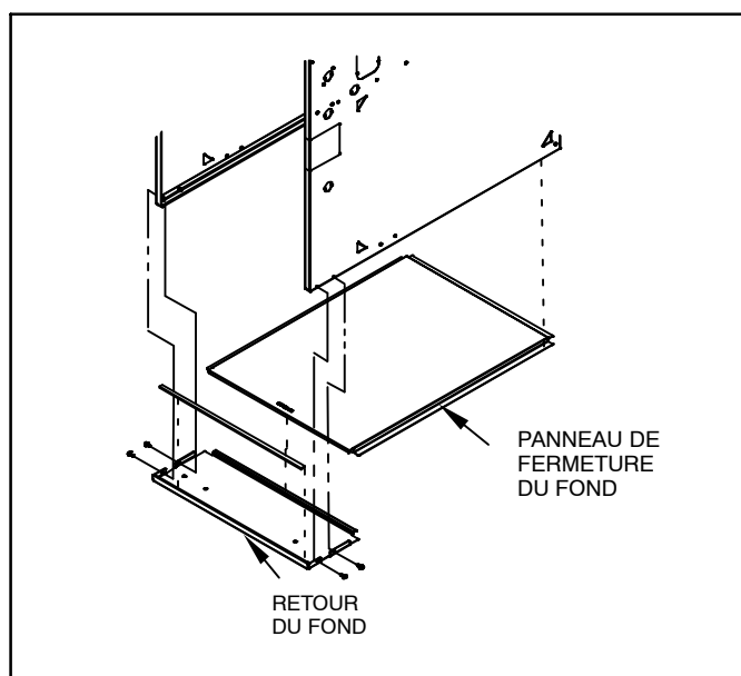
Figure 23 – Retrait du panneau de fermeture du fond
