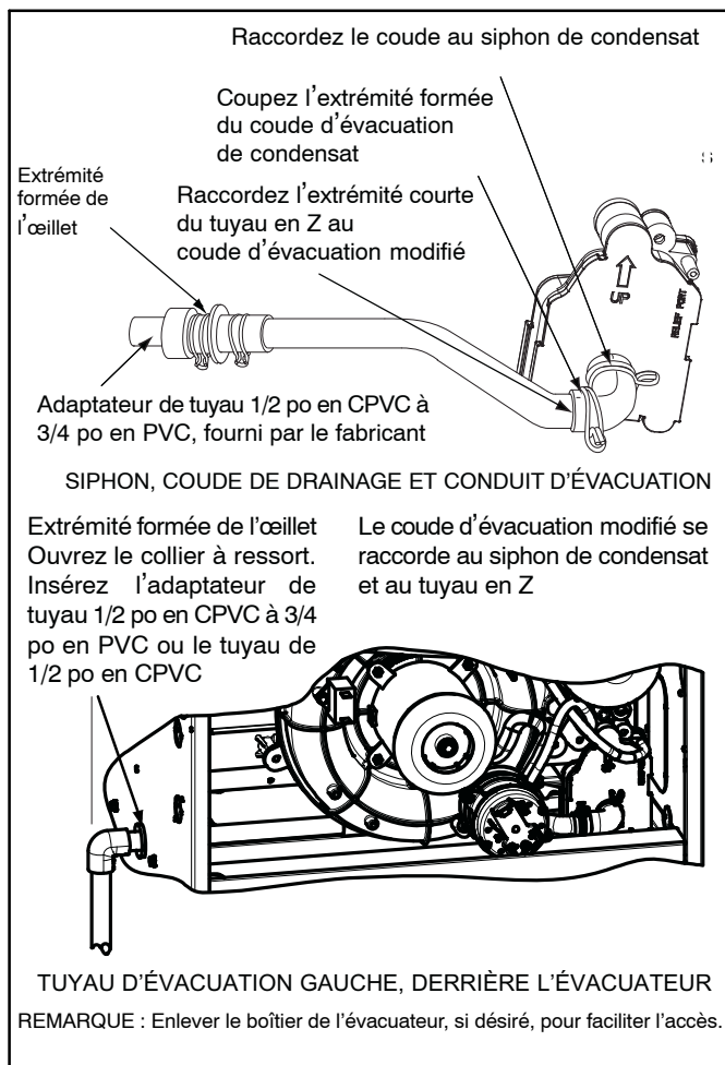
Figure 17 – Raccordement et acheminement du siphon d'évacuation (l'apparence peut varier)
